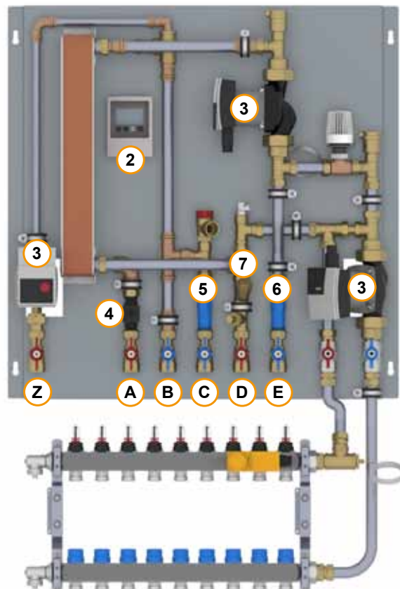
Frischwasserwohnungsstation TWWSe+Z+HKR
